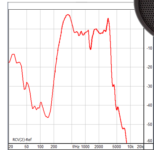
Lautsprecherfrequenzgang über TETRA Funk
