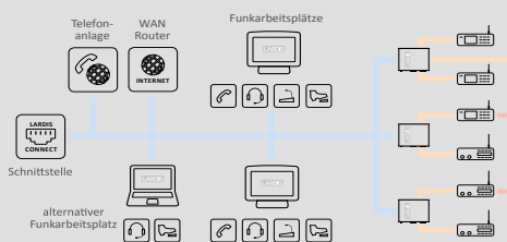
Beispiel ELW Systemaufbau mit LARDIS
